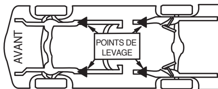
Cadre avant
