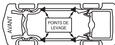
Cadre périphérique
