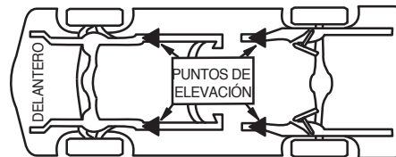
Chasis auxiliar
